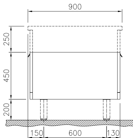
Zij aanzicht
